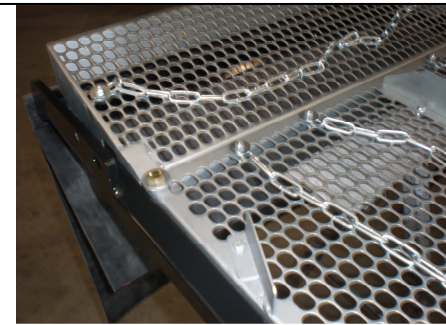
Obersiebrahmen mit hochgestellter Verlängerung + 18x22mm Langloch-Siebe + Ketten AF 1680 -7140
